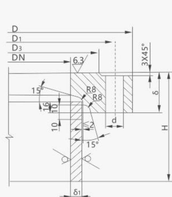
平密封面法兰
