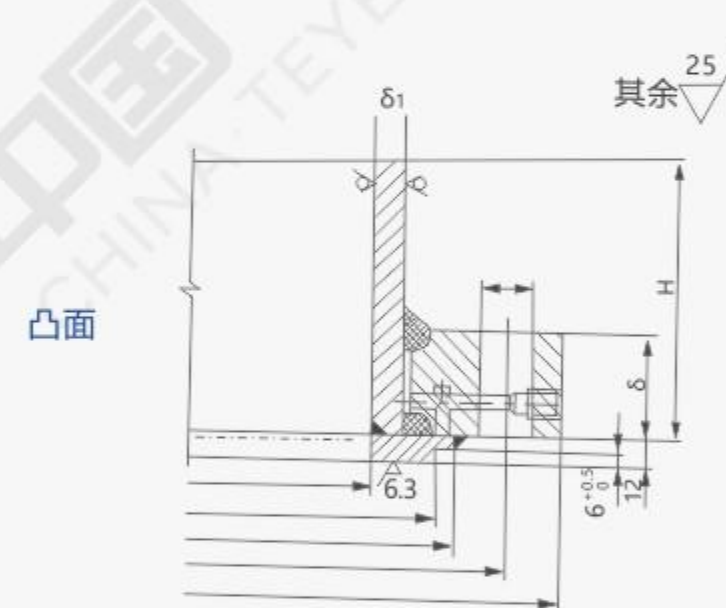
衬环平密封法兰 NB/T 47022-2012(JB/T 4702)
